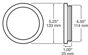
PM-B426-18 grommet
