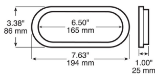
PM-B421-18 grommet
