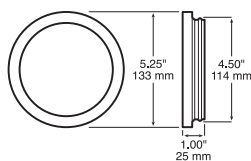
PM-B426-18 grommet
